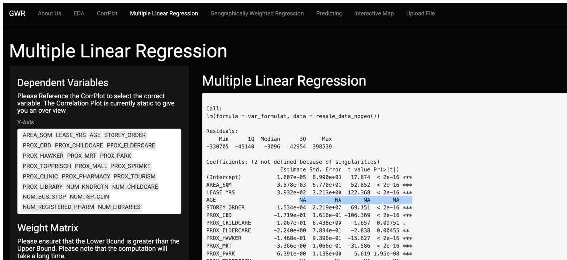
Fig. 4. MLR Tab
